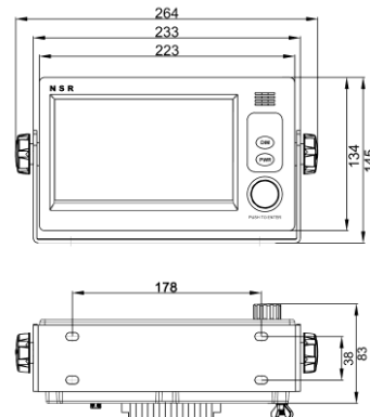
DISPLAY UNIT
